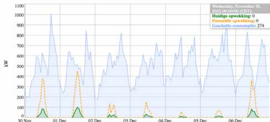
Stroomverbruik en stroomopwekking uit zonnepanelen op Sporenburg in eerste week van december
